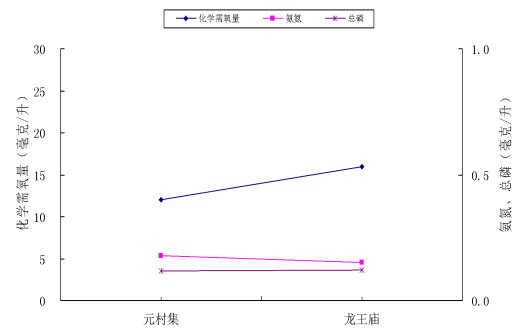
图14 2月卫河主要污染因子沿程变化
