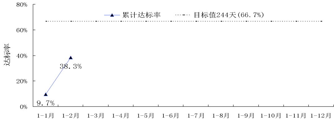
图2 2020年濮阳市环境空气累计达标情况
