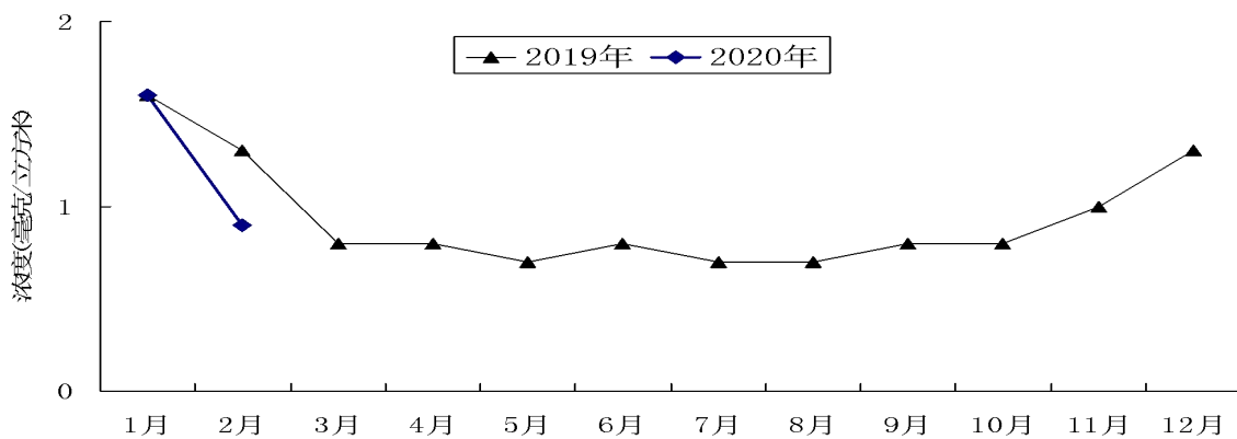
图6 濮阳市环境空气 NO 2 月均浓度走势图
