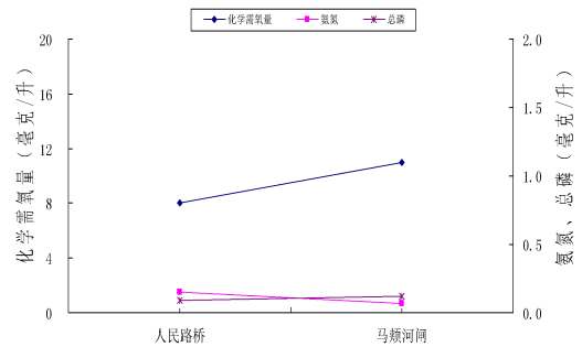
图12 2月濮水河主要污染因子沿程变化
