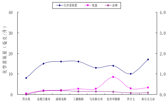
图11 2月马颊河主要污染因子沿程变化
