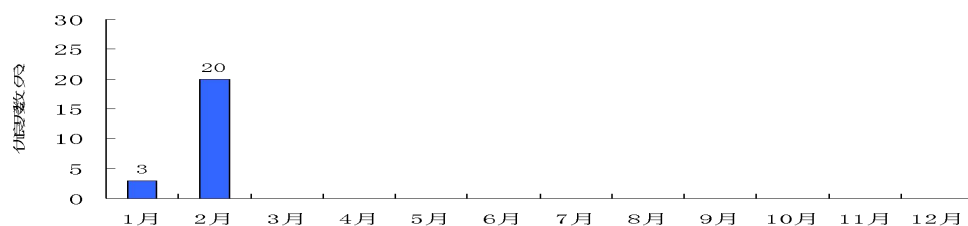
图 1 2020 年濮阳市环境空气优良天数情况
