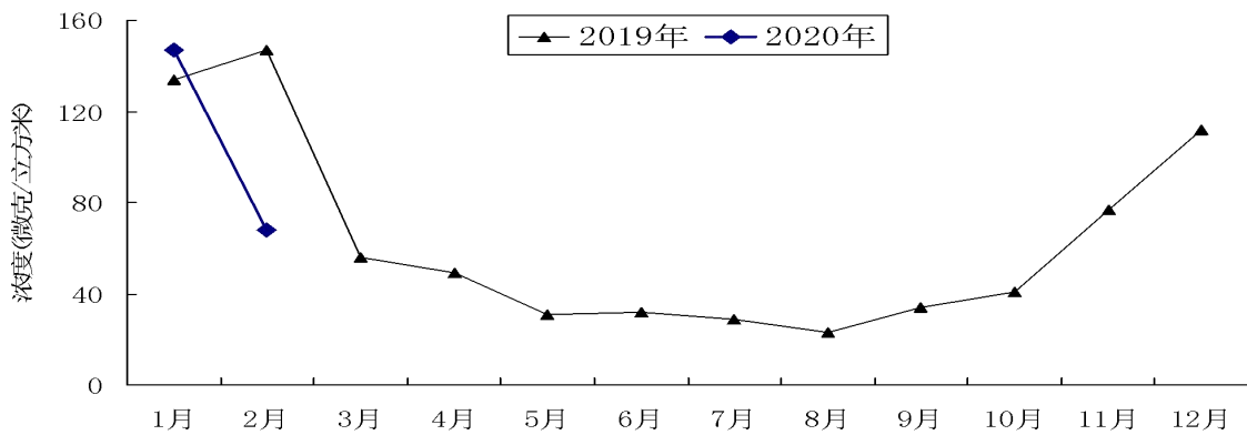
图4 濮阳市环境空气 PM 2.5 月均浓度走势图
