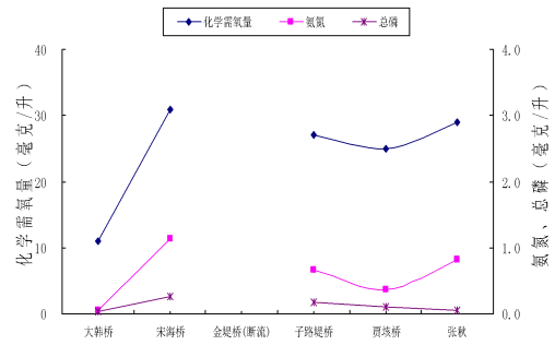
图10 2月金堤河主要污染因子沿程变化
