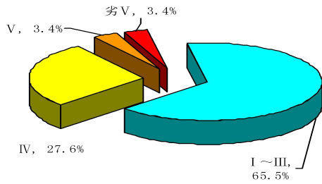
图9 2月主要河流断面水质类别比例
