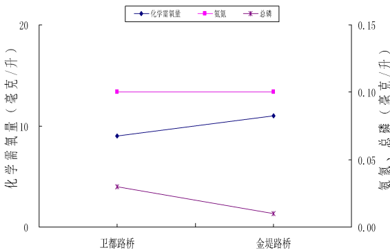
图13 2月卫都河主要污染因子沿程变化
